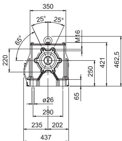
Flangia Riportata Bride modulaire
