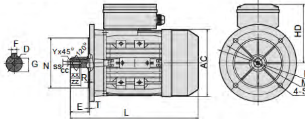
IMB5
