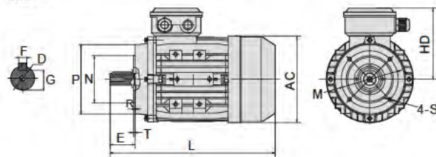
IMB14
