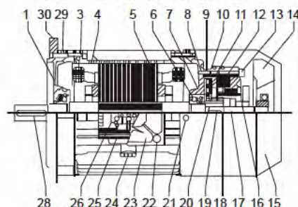
MSEJ Brake Motors B5 132~160
