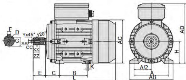
IMB3
