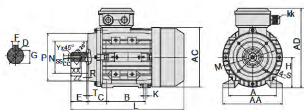
IMB34
