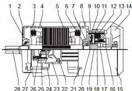
MSEJ Brake Motors B3 63~112
