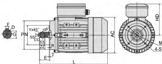
IMB14
