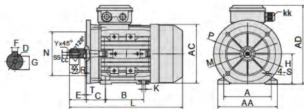
IMB35
