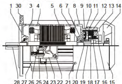
MSEJ Brake Motors B5 63~112
