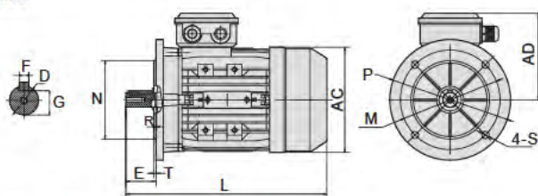
IMB5
